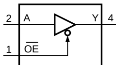
图 1 逻辑符号
