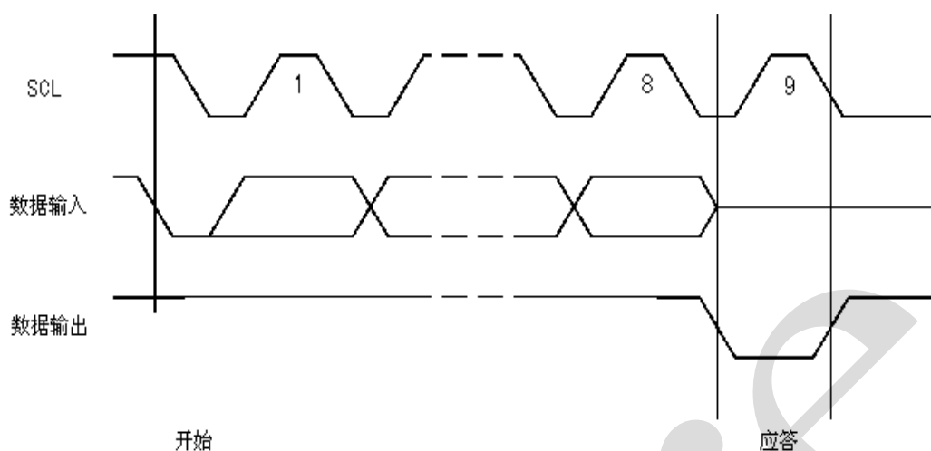
图 7、输出响应
