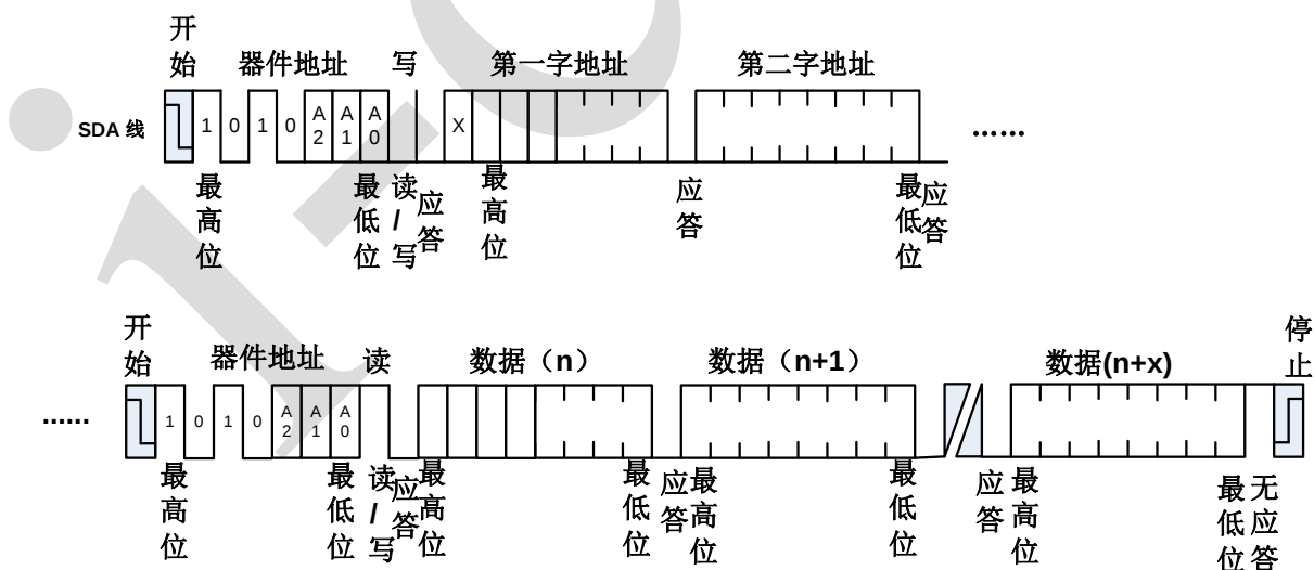
图 12、顺序地址读操作
