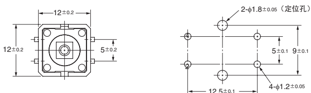
印刷基板加工尺寸（参考） （TOP VIEW） （印刷基板厚度 t=1.6 ）
