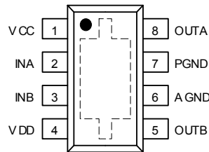
ESOP-8
