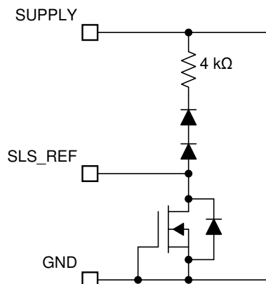
图 7-23. SLS_REF Pin
