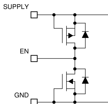
图 7-14. EN Pin
