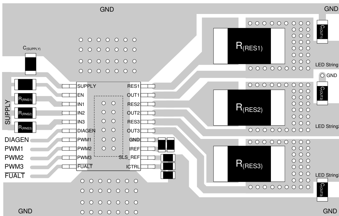
图 10-1. TPS92633-Q1 Example Layout Diagram
