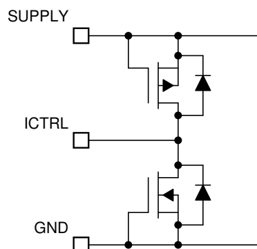
图 7-18. ICTRL pin
