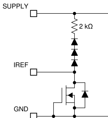
图 7-22. IREF Pin
