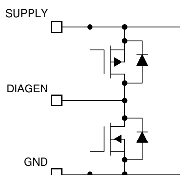
图 7-16. DIAGEN Pin
