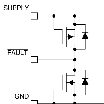
图 7-17. FAULT Pin
