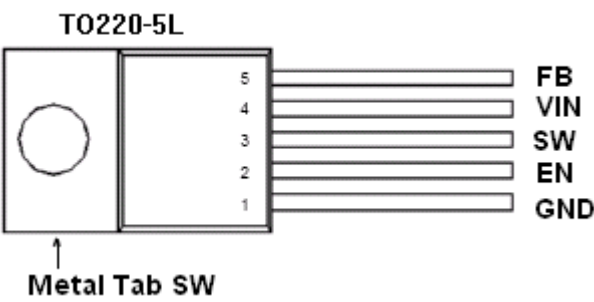
图 2. XL6012 引脚配置
