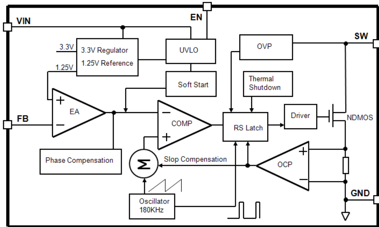
图 3. XL6012 方框图
