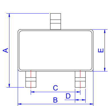
SOT-23
