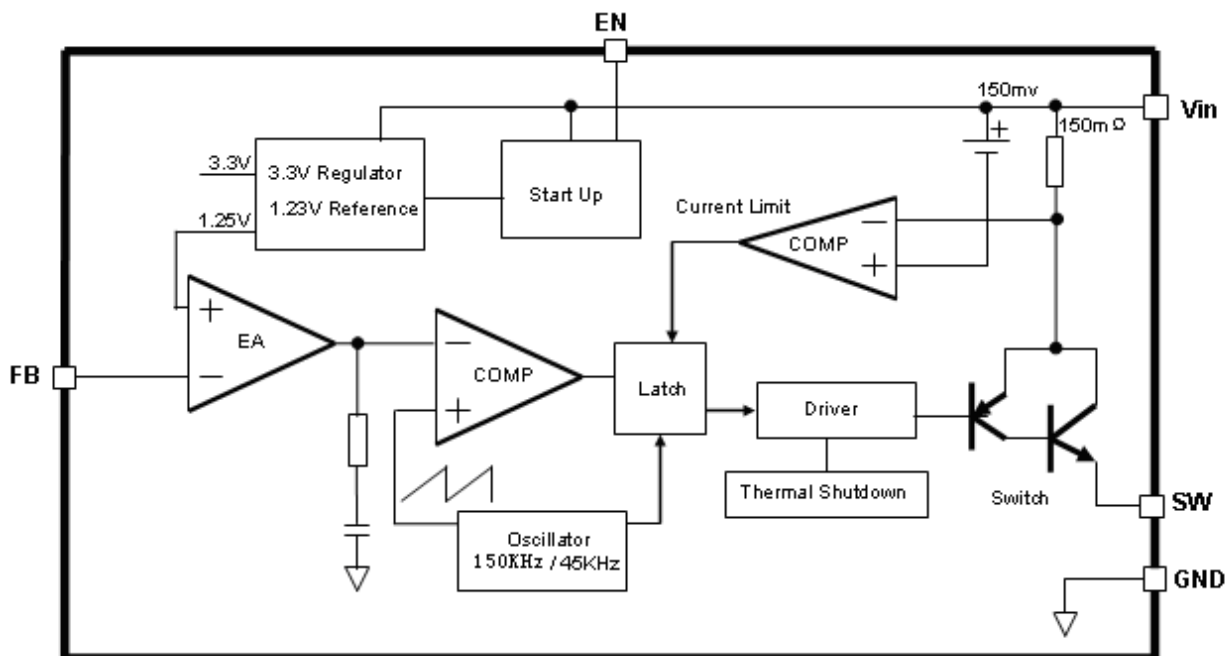
图 3. XL7015 方框图
