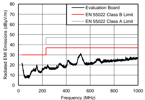
辐射发射图
