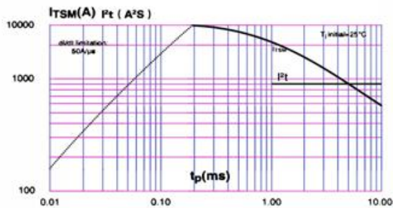
6、 I_{TSM}-t_p 、 I^2t-t 曲线
