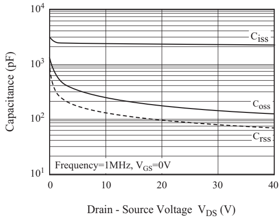
Fig 9. C - V_{DS}
