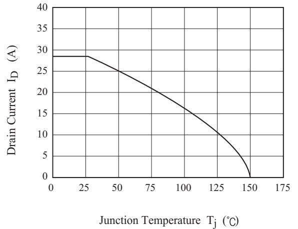
Fig8. I_D - T_j
